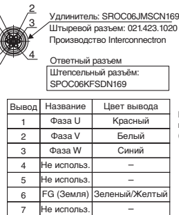
Назначение выводов и параметры разъема линейного серводвигателя
